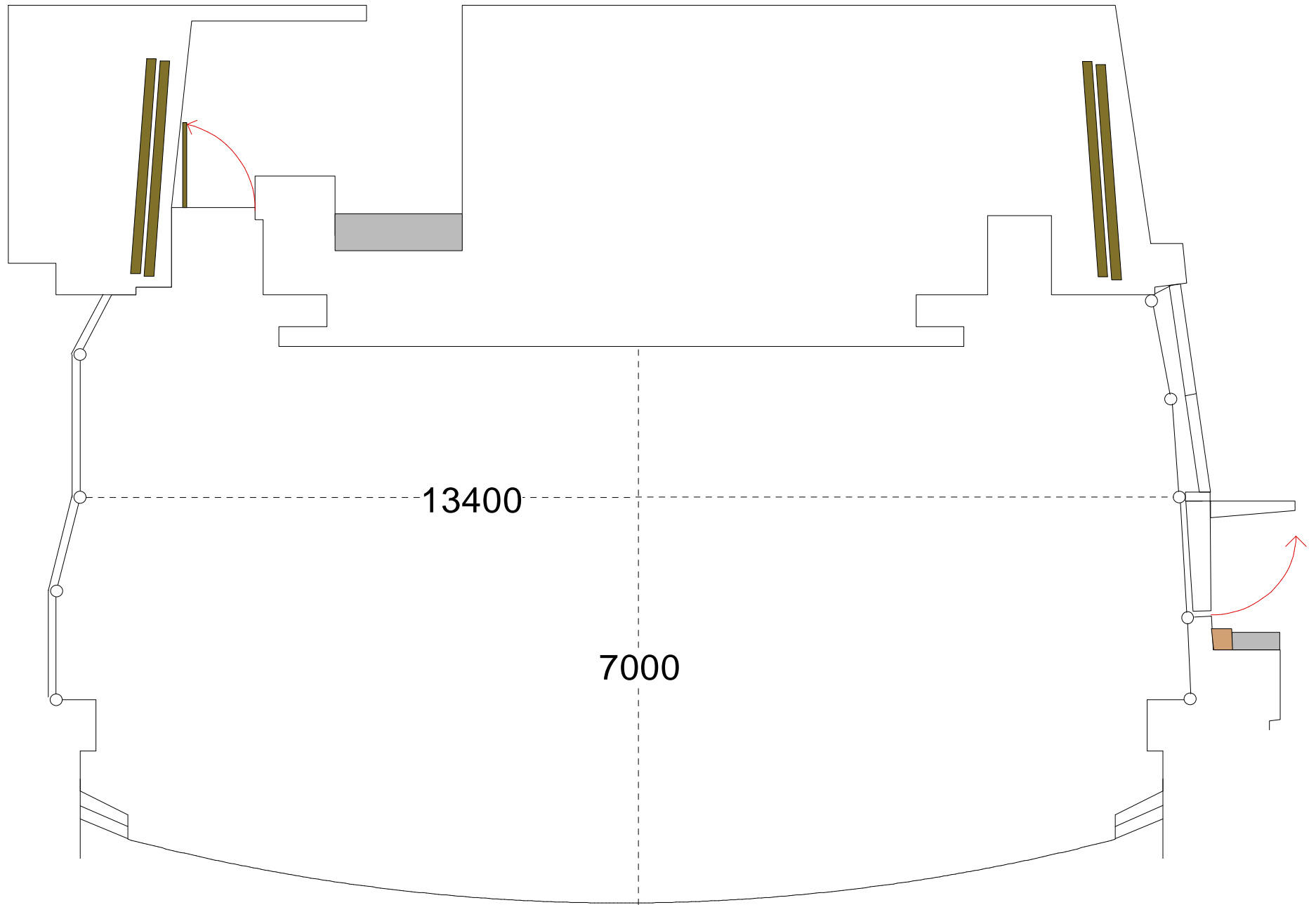
横浜みなとみらいホール 小ホール平面寸法図
