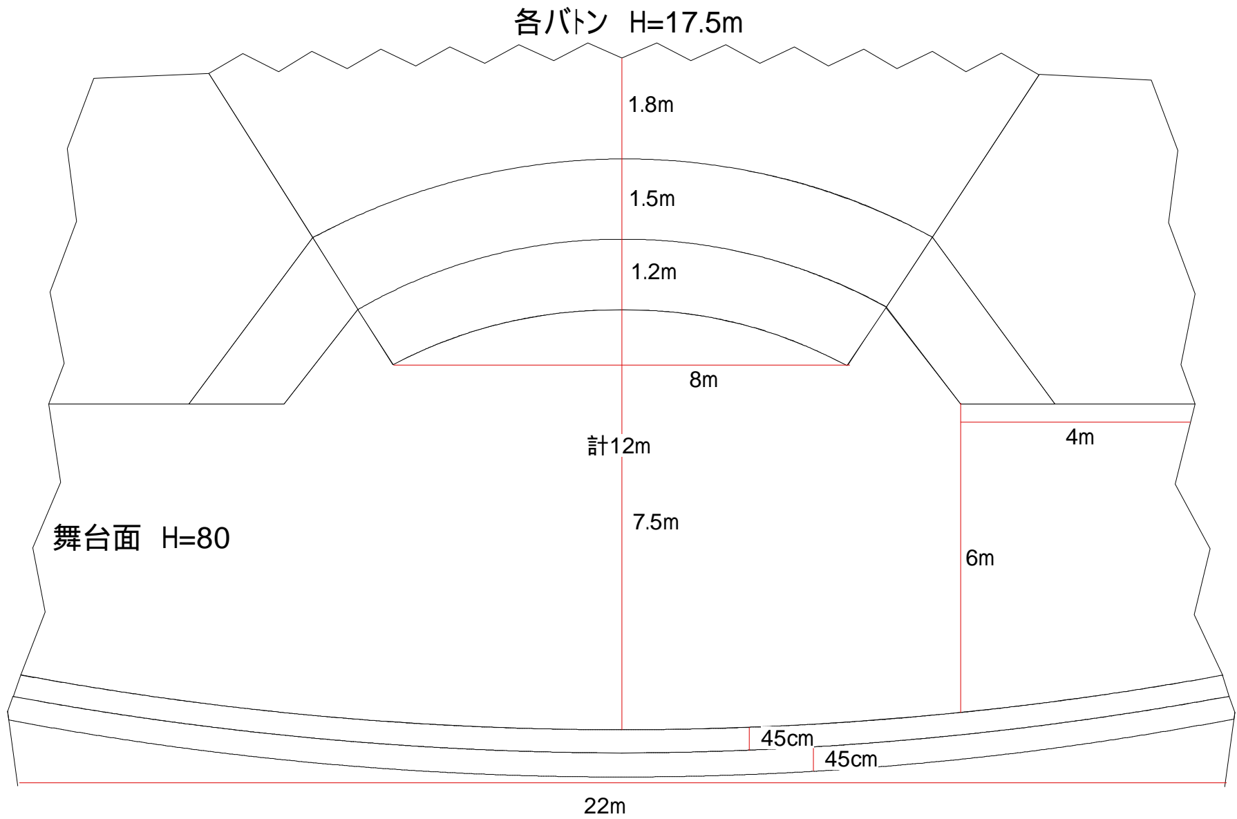
横浜みなとみらいホール 大ホール寸法図
